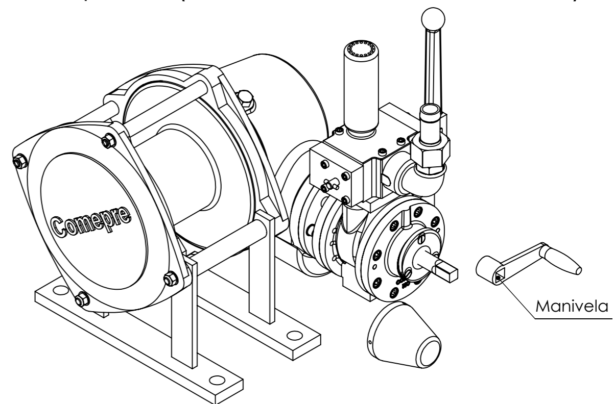
Guincho com motor a ar G050 Tipo G050 0MP5-02 com dispositivo manual acoplado. (Na falta de ar, usar manivela)
