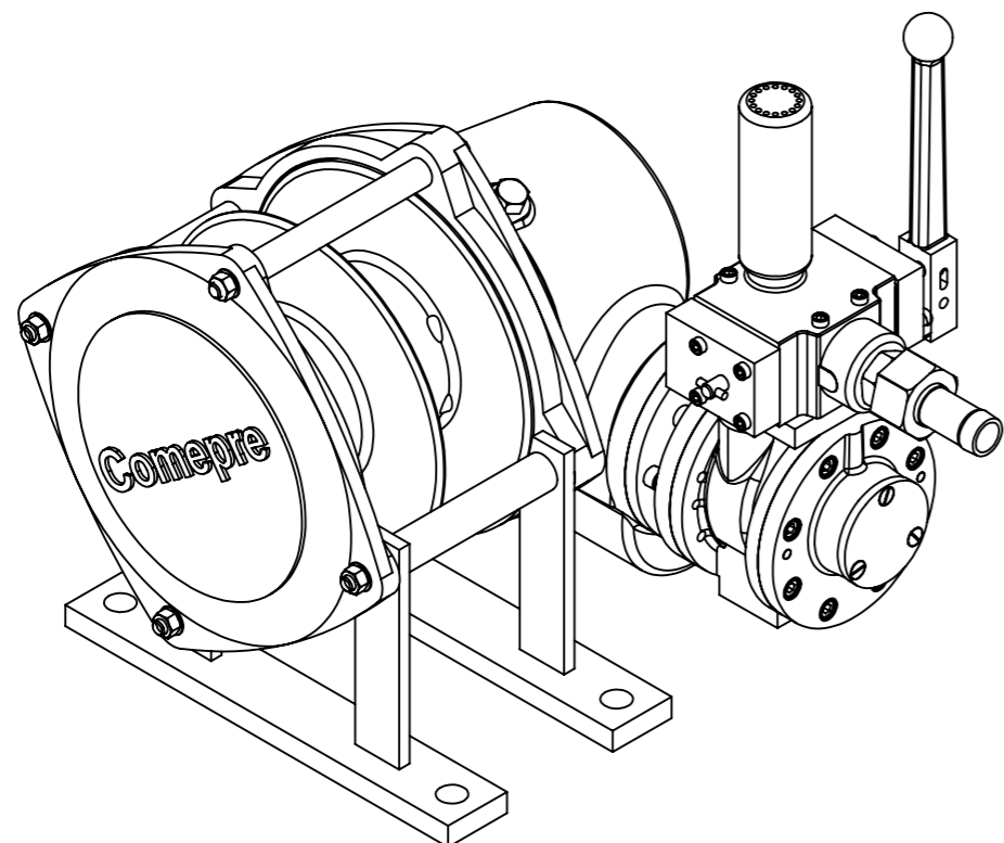
Guincho de tambor duplo com motor a ar G050 Tipo G050 0MP5-11 comando manual acoplado
