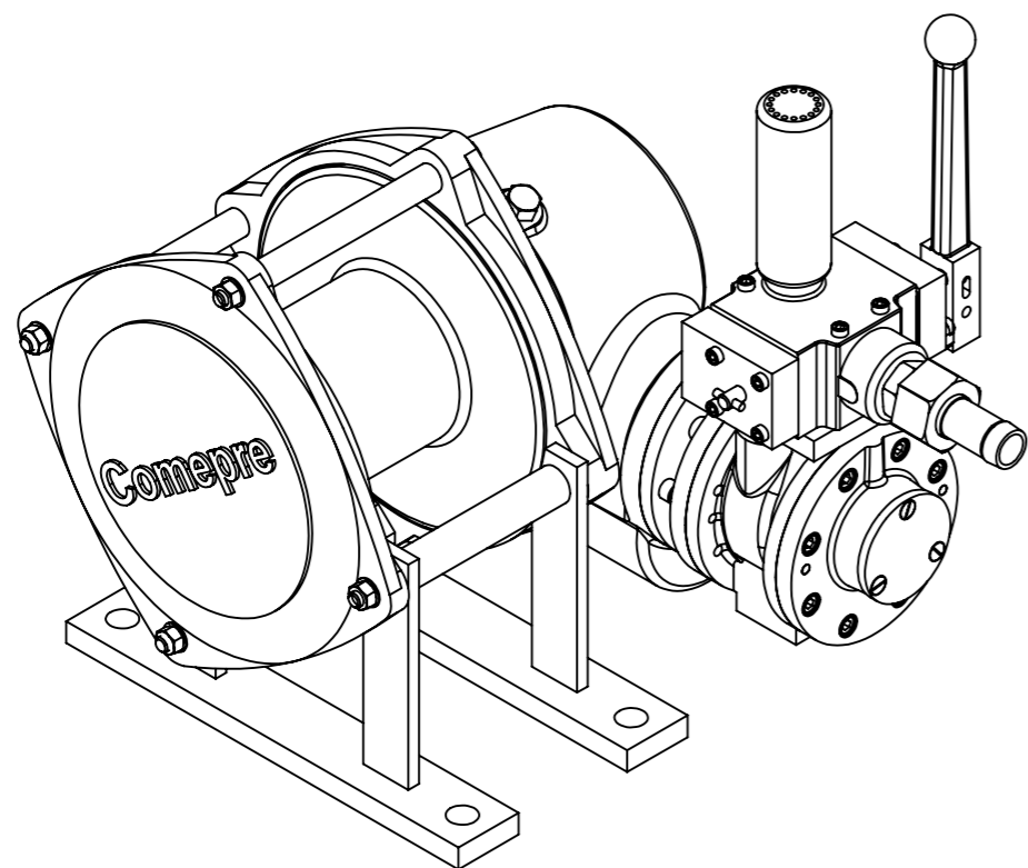
Guincho de tambor duplo com motor a ar G050 Tipo G050 0MP5-11 comando manual acoplado
